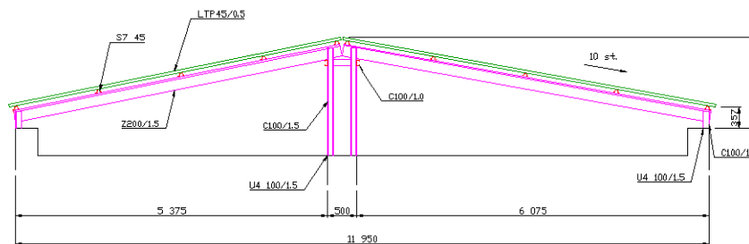
podélný systém (zde dvojtrakt)
