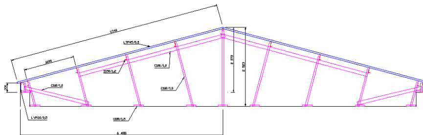
příčný systém (modul např. 3,6 m)
